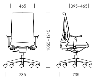
Drehstuhl, Rücken Standard Siège de bureau, dossier standard
