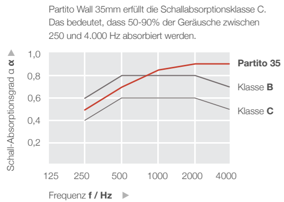
D1013 | PARTITO WALL (AP20), QIVI FREISCHWINGER (TR12/AT16/MESH 05)
